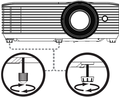
Регулятор наклона
